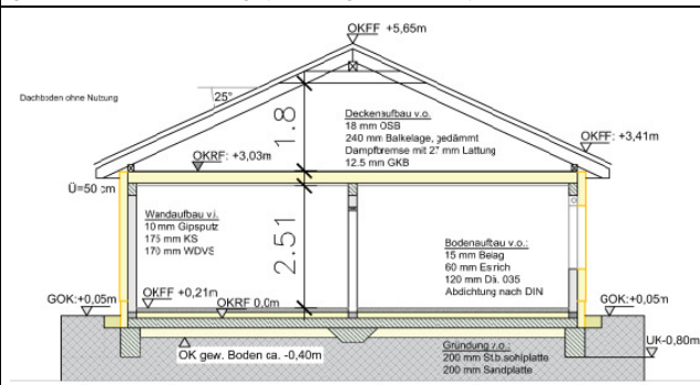
Systemschnitt (© Ing.-Büro Brinkmann 2018)
